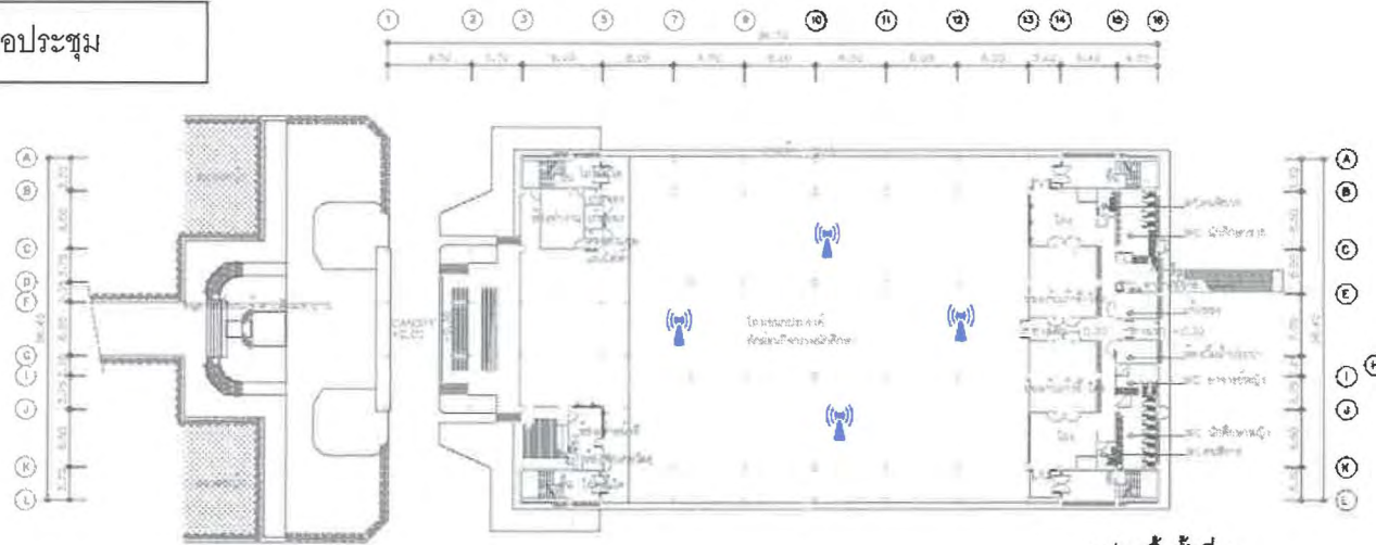
แปลนพื้นที่ 1 (อาคารหอประชุม)
