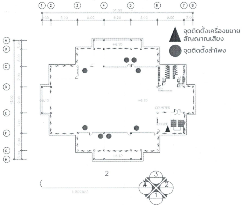
แผนผังการติดตั้งเครื่องเสียงและลำโพง
