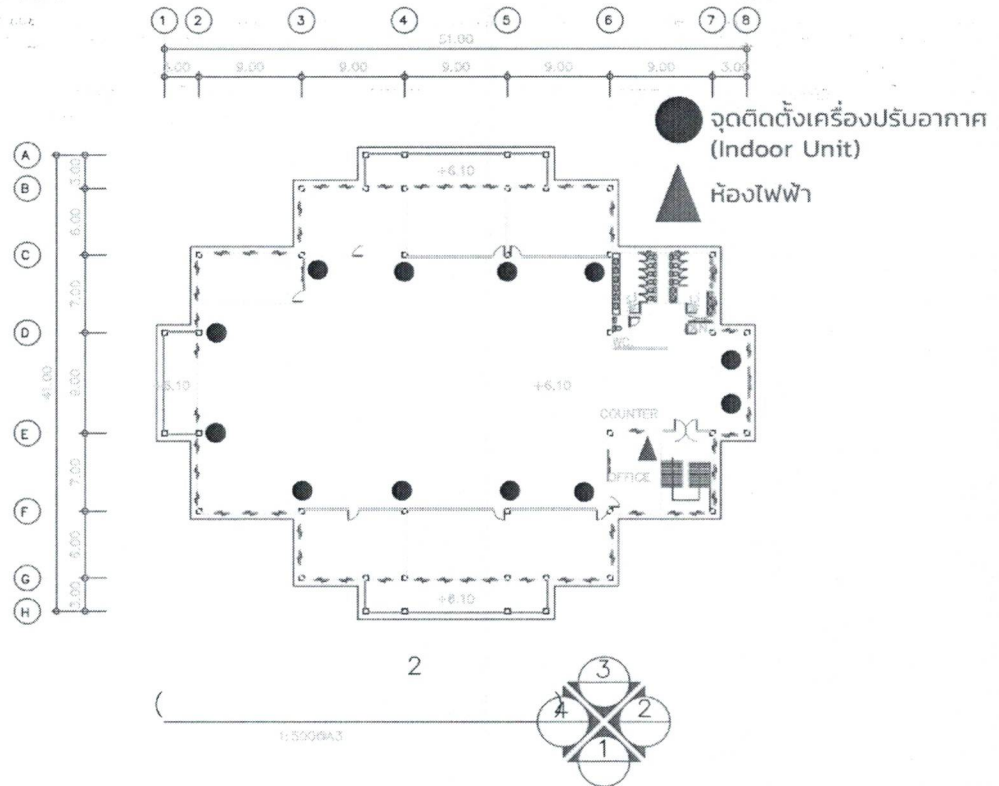
แผนผังการติดตั้งเครื่องปรับอากาศ
